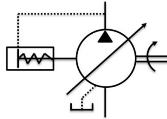
油壓記號 SYMBOL
